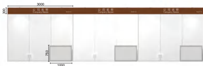
展位正立面图
